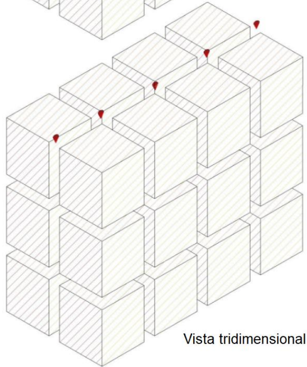
Figura 4.19: Leiaute de chuveiros automáticos para estrutura-suporte de fileira dupla – Leiaute “H” - Opção # 2.
