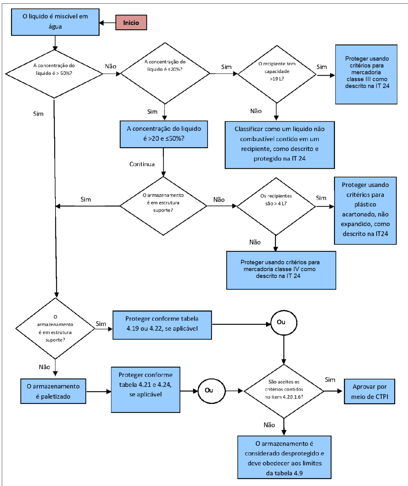
Figura 4.4: Árvore de decisão para o critério de proteção contra incêndio para líquidos inflamáveis e combustíveis miscíveis em água contidos em recipientes não metálicos.
