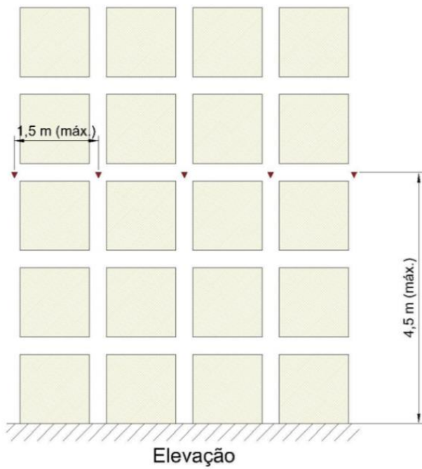
Figura 4.19: Leiaute de chuveiros automáticos para estrutura-suporte de fileira dupla – Leiaute “H” - Opção # 2.
